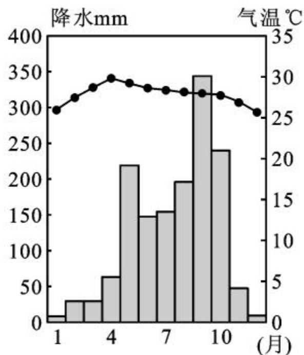
曼谷多年平均各月气温和降水量
